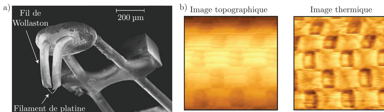
Figure 1 – a) Image au microscope à balayage électronique de la micro-pointe Wollaston [1]. b) Images topographique et thermique obtenues sur un damier micrométrique constitué de deux matériaux de conductivités thermiques différentes [2].
